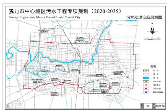
给排水工程项目的规划设计
